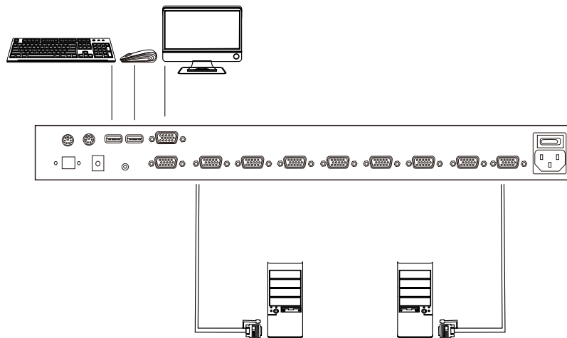
联机示意图
